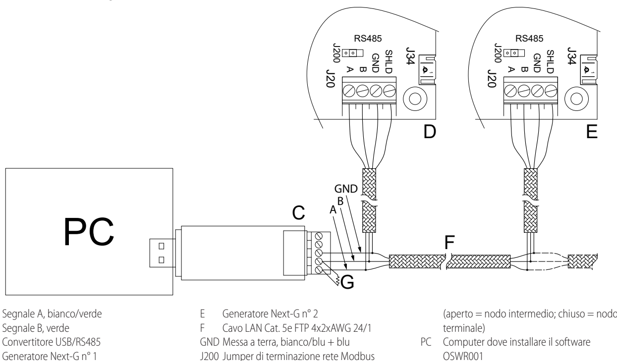
Figura 6.1 Schema di collegamento rete Modbus
